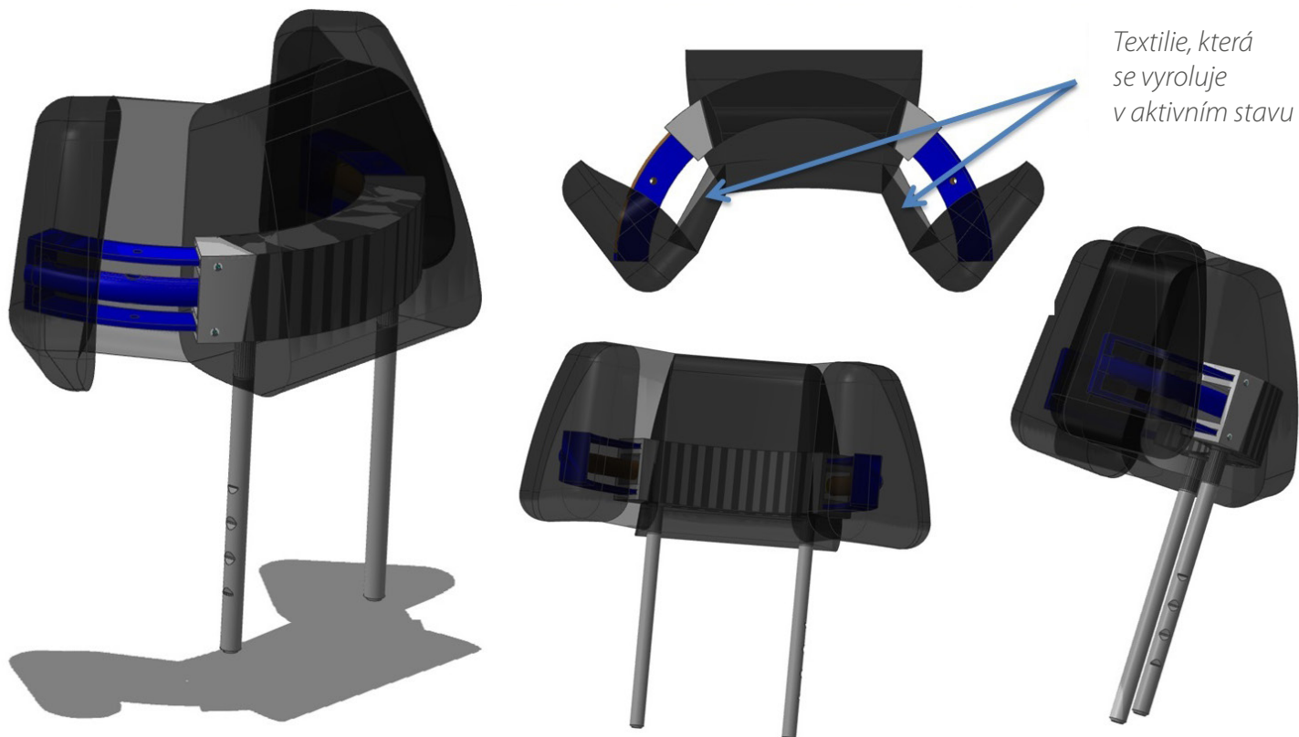
model aktivní opěrky hlavy s inovativním systémem
