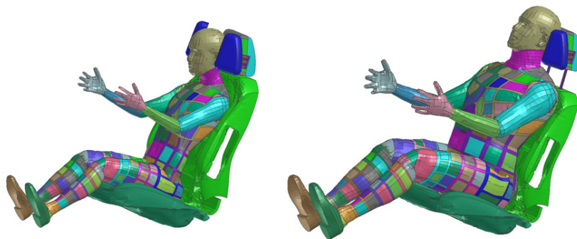
testování aktivní hlavové opěrky - vliv antropometrie řidiče
