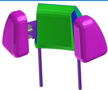
barevné znázornění hlavních částí aktivované opěrky hlavy
